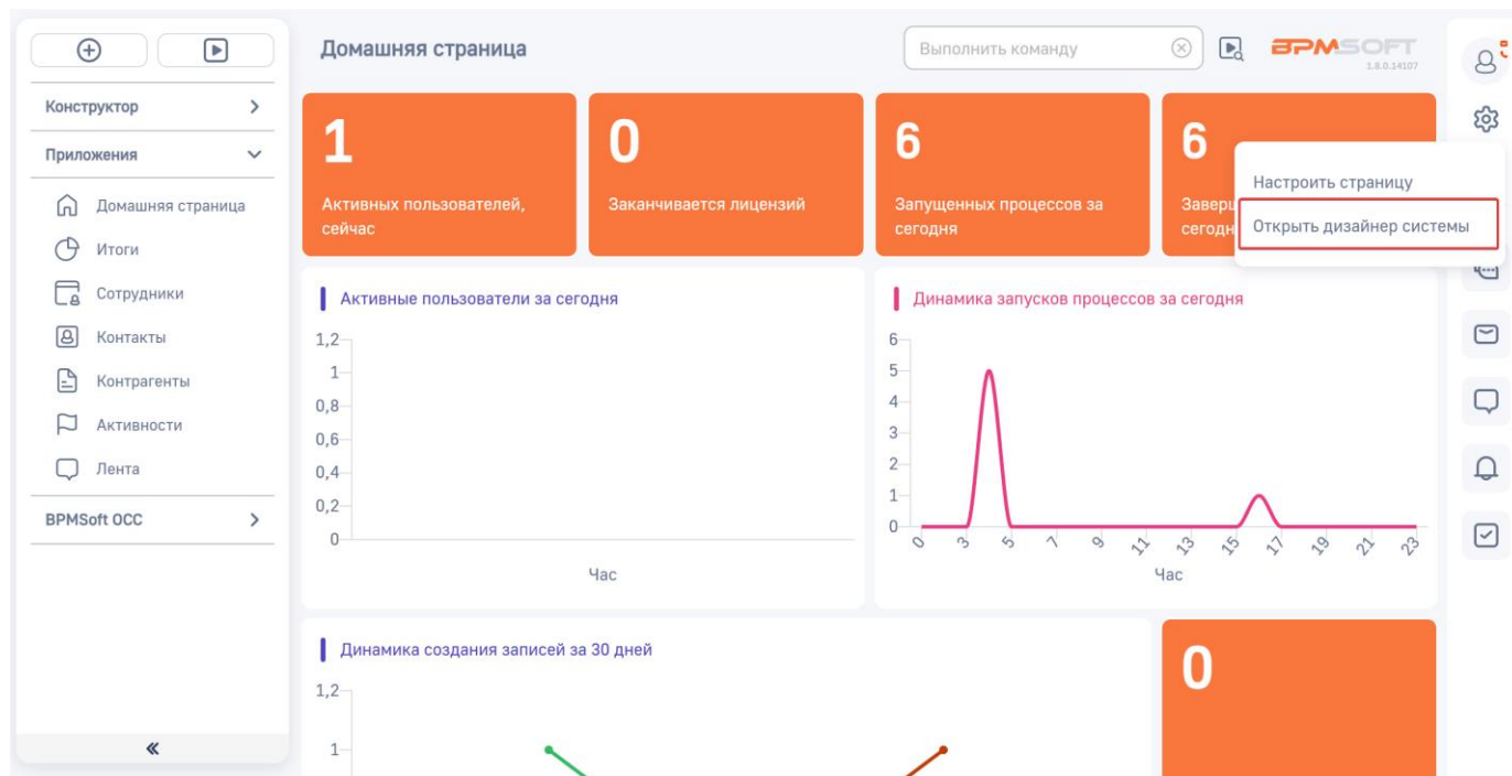
Рисунок 1 – Главный экран
