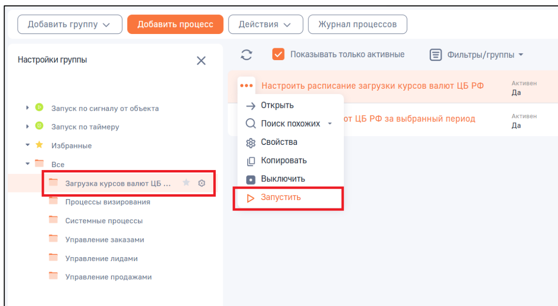
Рисунок 15 – Запуск процесса «Настроить расписание загрузки курсов валют ЦБ РФ»
