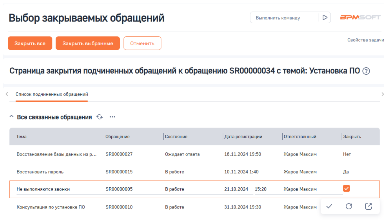
Рисунок 7 — Выбор подчиненных обращений для закрытия
