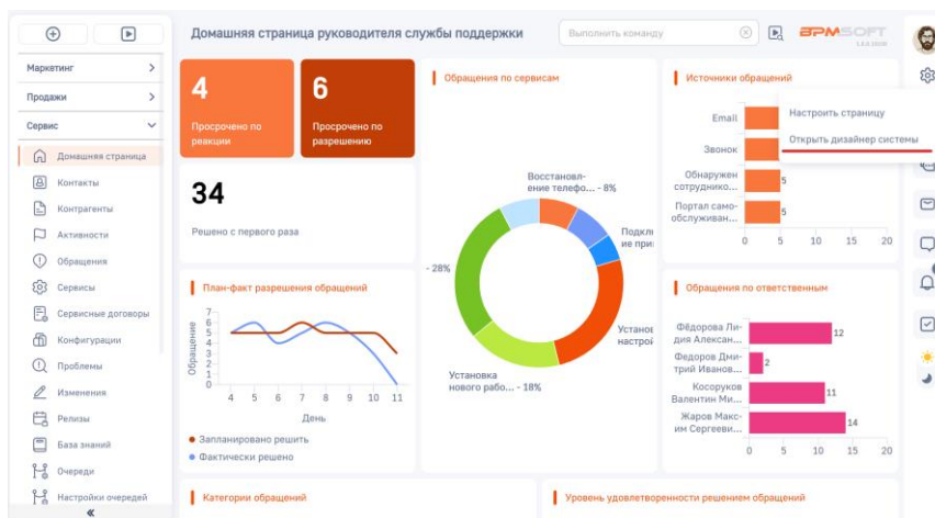
Рисунок 1 – Главный экран
