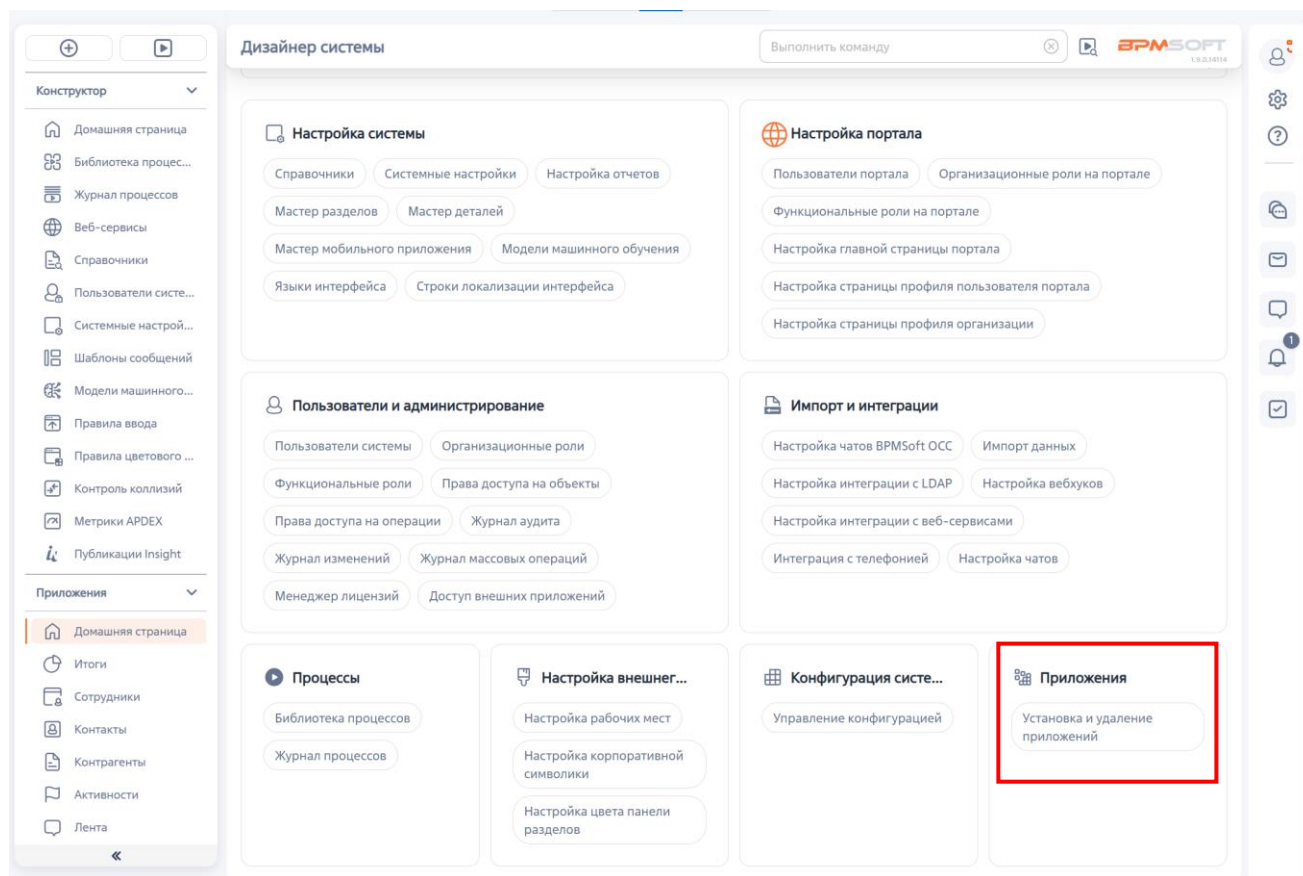
Рисунок 4 – Дизайнер системы
