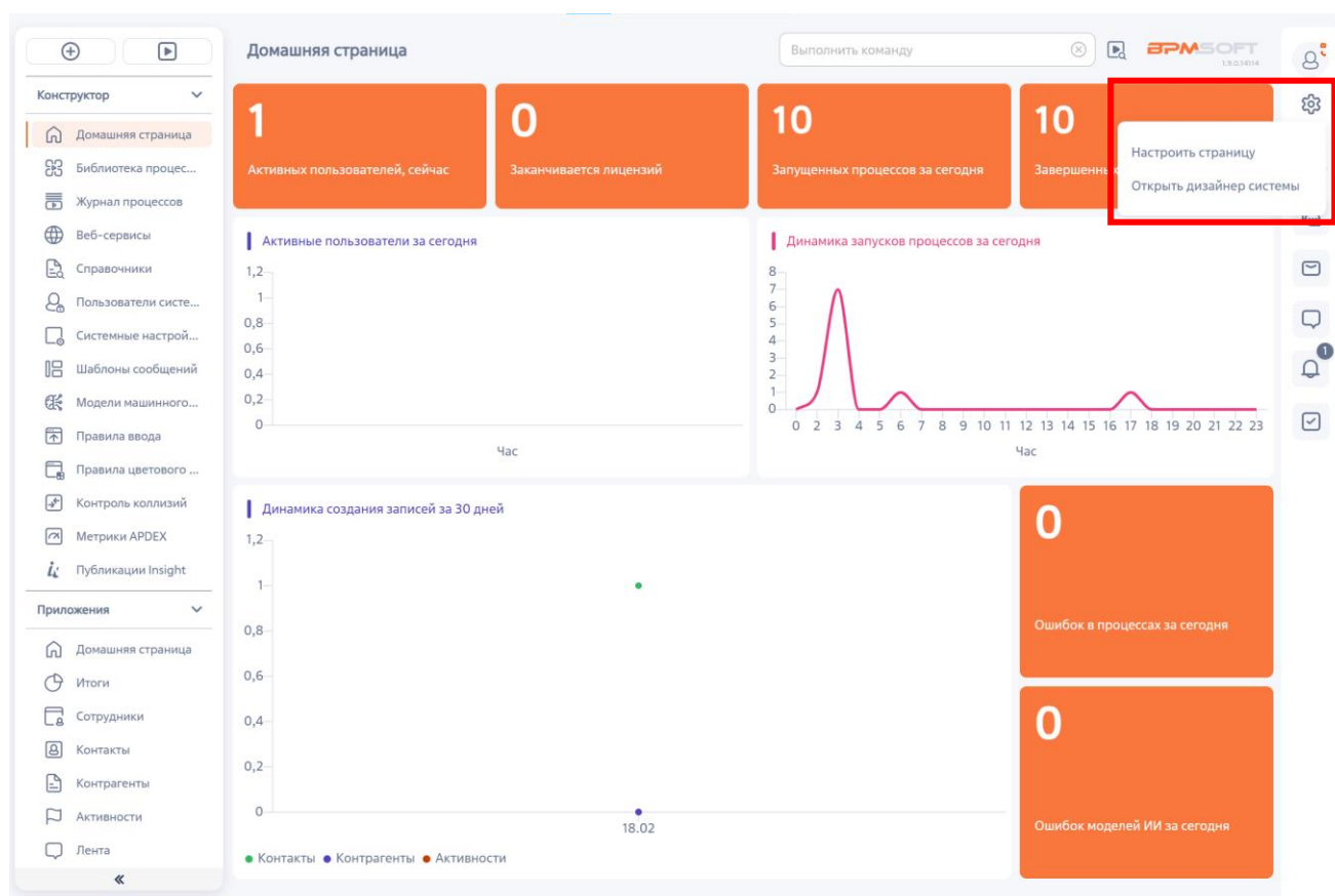
Рисунок 1 – Главный экран
