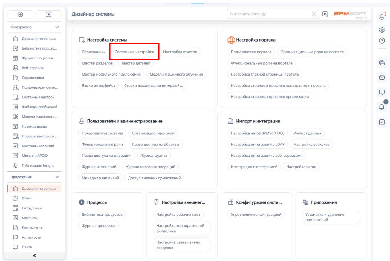
Рисунок 2 – Системные настройки
